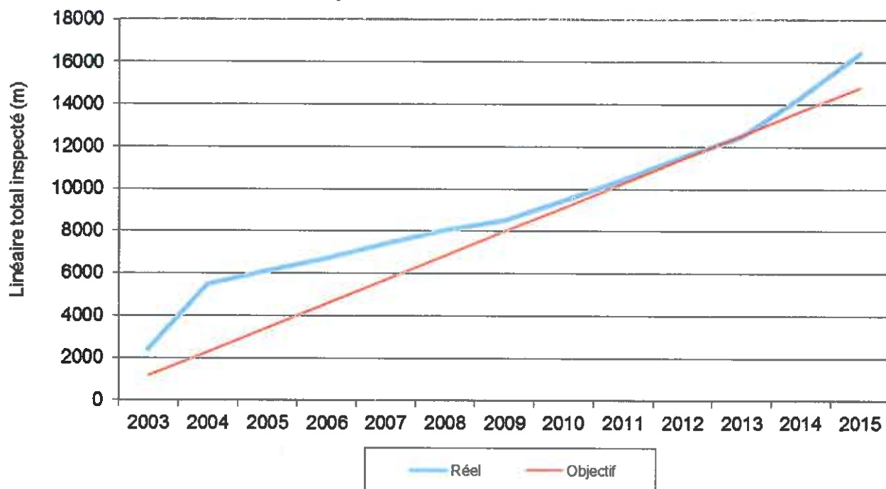
Inspection télévisée des collecteurs
