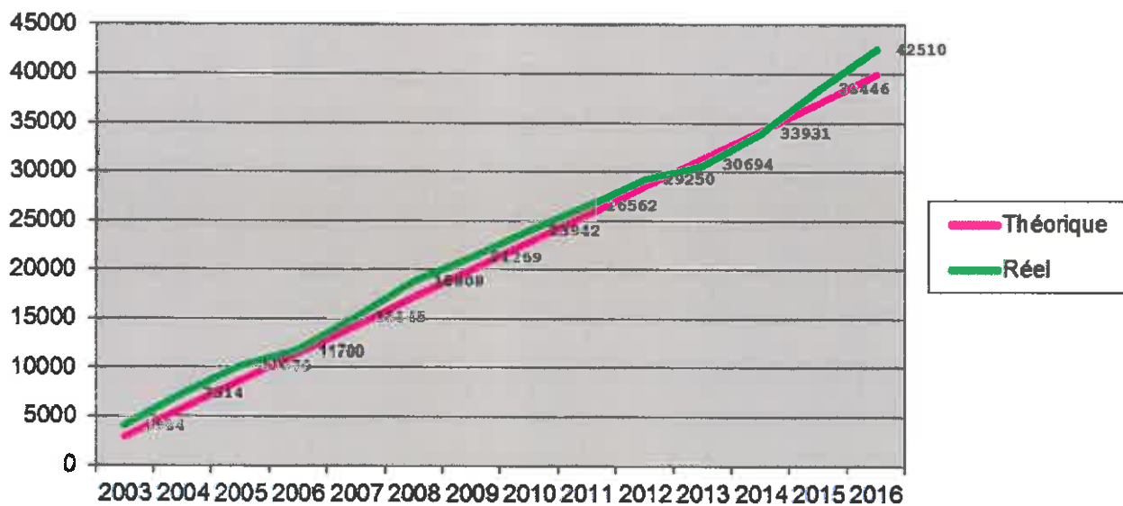
Courbe du linéaire de curage
