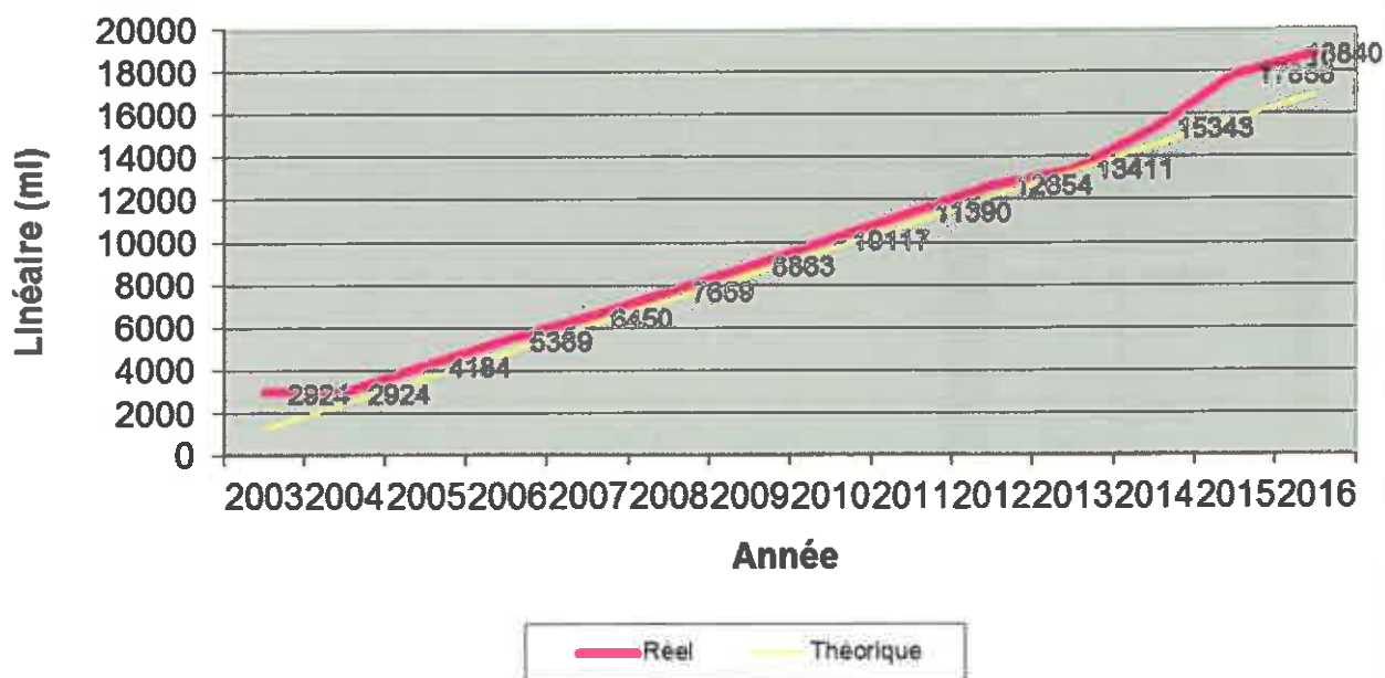
Inspection télévisée des collecteurs EU
